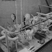
Газораспределительное устройство.
