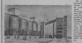
На снимке — автоматизированный бетонный завод, недавно введенный в строй на строительстве Кузнецкого гидроэлектростанции. Он сооружен с учетом последних достижений отечественной науки и техники. Чтобы выложить и затвердеть бетон, оператору достаточно нажать кнопку. В сутки предприятие выдает две тысячи кубометров бетона. Для приготовления такого количества бетона ручным способом потребовалось бы 1500 рабочих, а автоматизированный завод обслуживают лишь 10 человек в смену.
