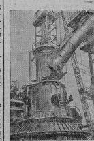
На снимке: монтаж узлов второй домненической печи комбината Карла Готвальда в Кучинце. Фото Чехословацкого телеграфного агентства.
