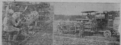
Машина для квадратной посадки рассады овощей. Сепараторная часть машины, сир на общий привод. Пресскавказ ТАСС
