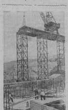
Тяжелая ССР. Строительством Кавказского гидроэлектростанции на реке Сур-Дарас. Из снимков монтажных работ. Фото В. Зайцева.
