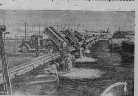
Современная в честь XX съезда партии, строители Горьковской гидроэлектростанции перенесли Восток 24 августа, являясь, чем предусматривалось графиком. Рукава Восток полностью перекрыты, и вода реки пошла через открытые проемы водосточной системы.
