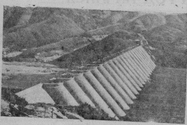
Китайская Народная Республика. Фольклорные водохранилища на реке Бянь (провинция Аньхуй). Его, емкостью—470 миллионов кубических метров воды. Фото агентства Синауа.
